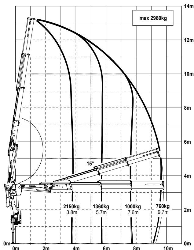
B (3段伸縮ブーム)
