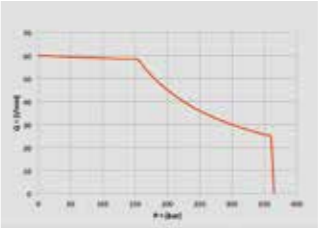
Leistungsregelung 15 [kW]
