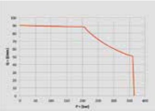
Leistungsregelung 30 [kW]
