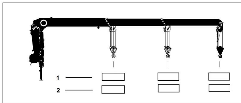
Рис.14: Табличка грузоподъемности (пример)
