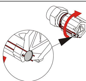
Рис.17: Расположение клапана аварийного останова на гидрораспределителе Danfoss (пример)
