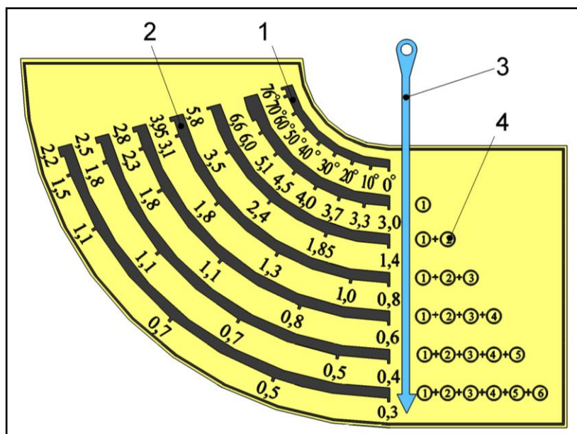
Рис.15: Указатель угла наклона стрелы (пример)
