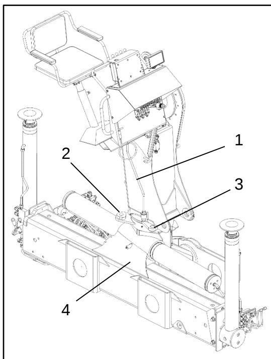
Рис.11: Фиксация колонны при управлении с колонны
