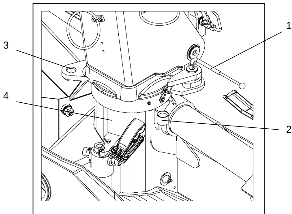
Рис.12: Фиксация колонны при управлении с нижнего пульта
