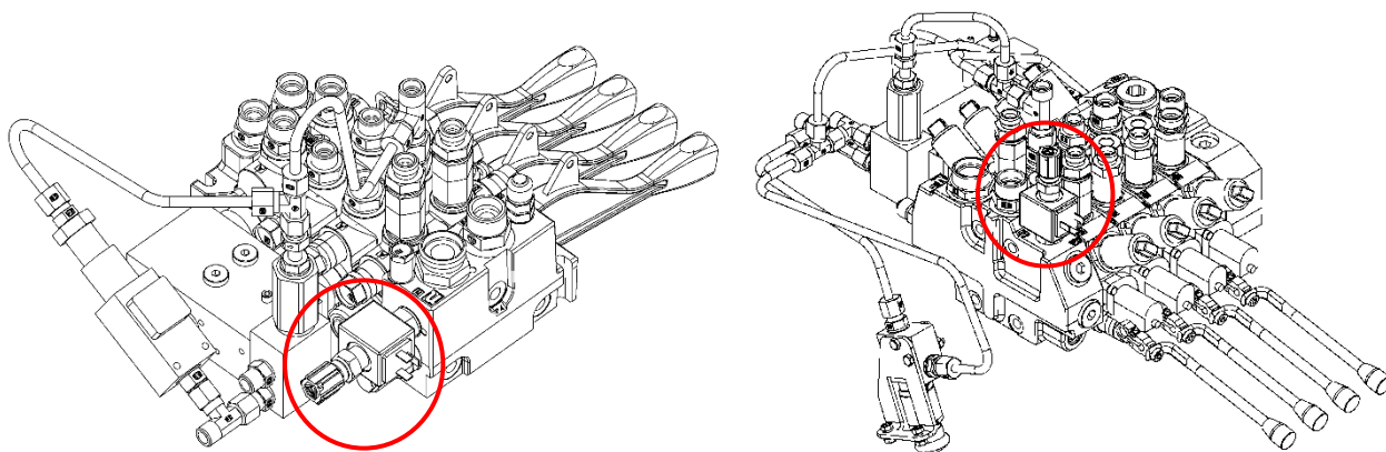
Рис.16: Расположение клапана аварийного останова на гидрораспределителях Nordhydraulik (пример)
