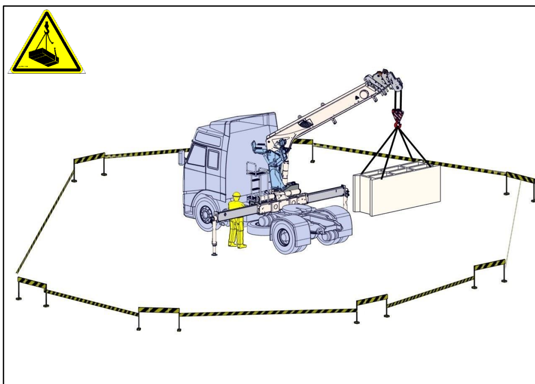
Рис.9: Огражденная опасная зона
