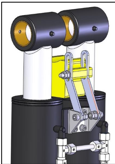
Рис.13: Транспортировочный упор стреловой системы
