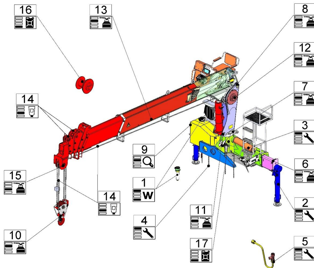
Рис.20: Схема обслуживания КУ (пример)
