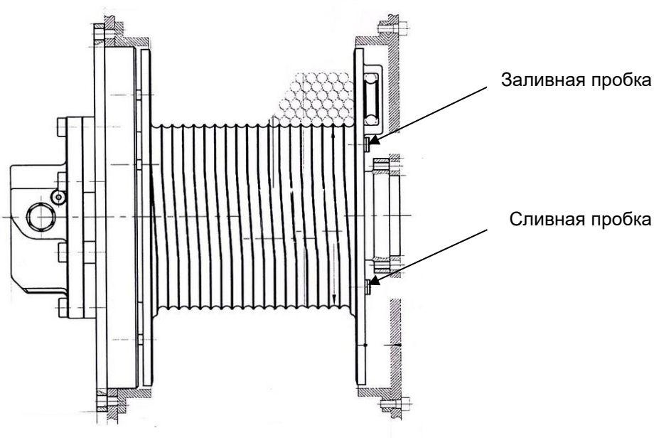
Рис.21: Лебедка с расположением сливной и заливной пробок на боковой (торцевой) поверхности барабана
