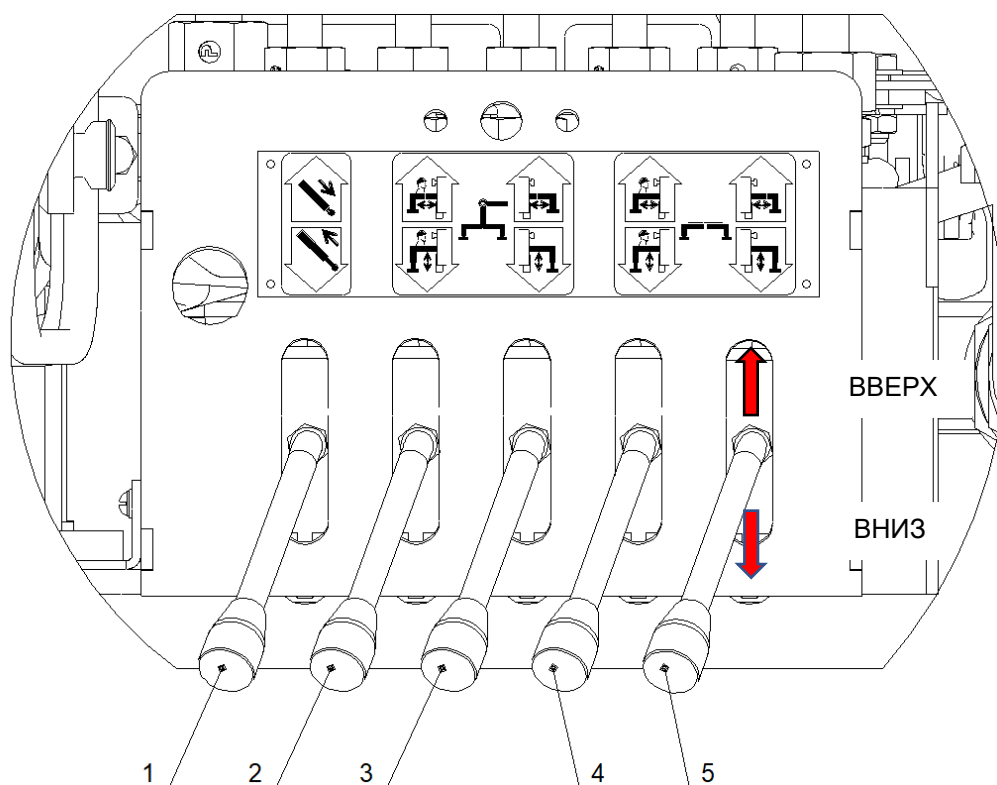
Рис.15: Панель управления со стороны гидрораспределителя аутригерами и опорными гидроцилиндрами КУ (пример)
