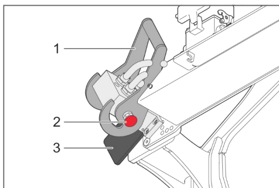
Рис.13: Быстросъемное соединение для гидравлического оборудования
