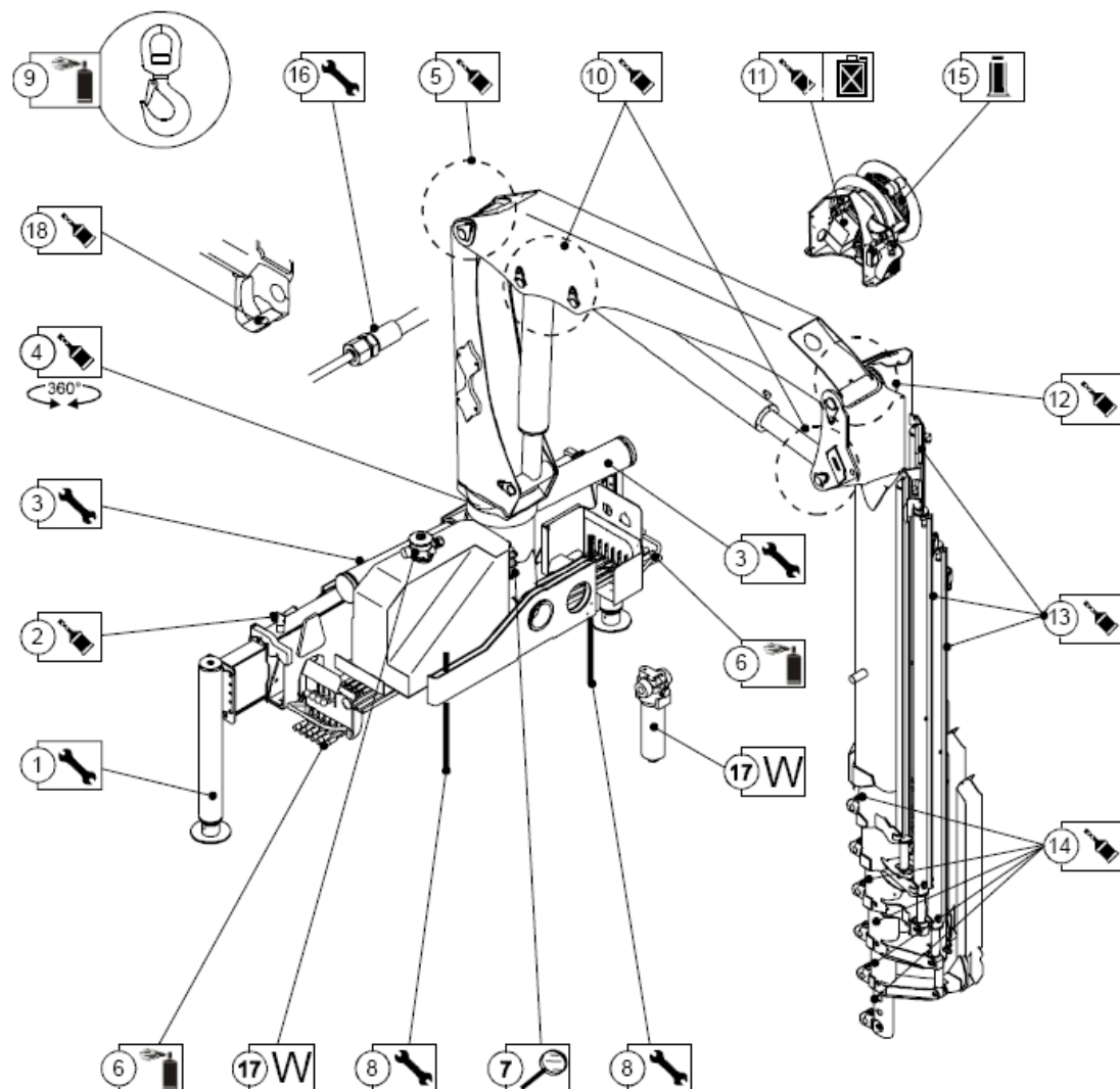
Рис.22: Схема обслуживания крановой установки
