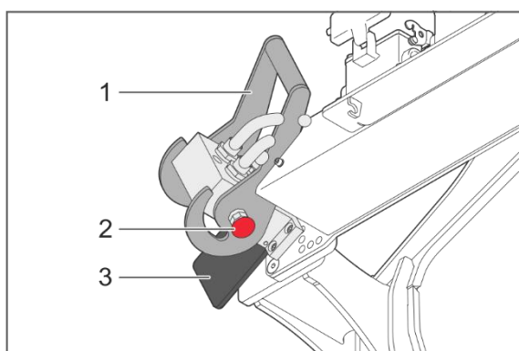
Рис. 13: Быстроразъемное соединение для гидравлического оборудования
