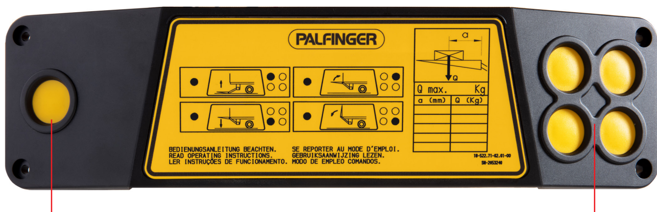
Bouton de commande à deux mains (EN ISO 13851)
