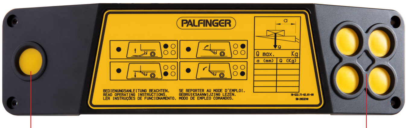
Safety two-hand operation button (EN ISO 13851)
