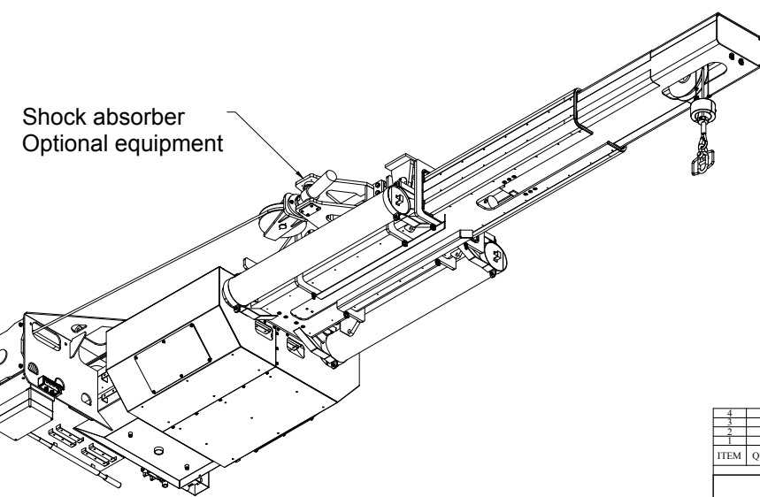
Isometric (1 : 25)
