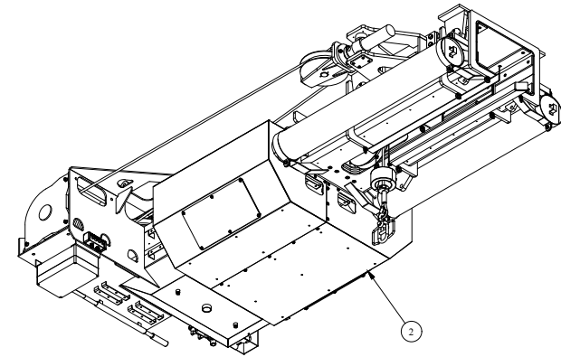
Isometric (1 : 25)
