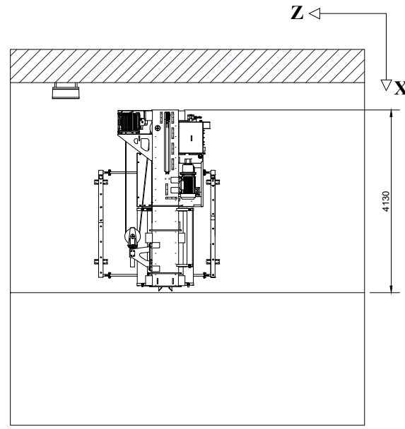
J-J (1 : 60)
